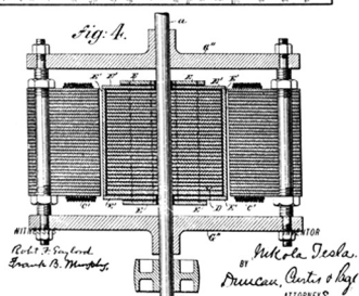
Slika 4. Elektromagnetski motor, patent br. 382279.
